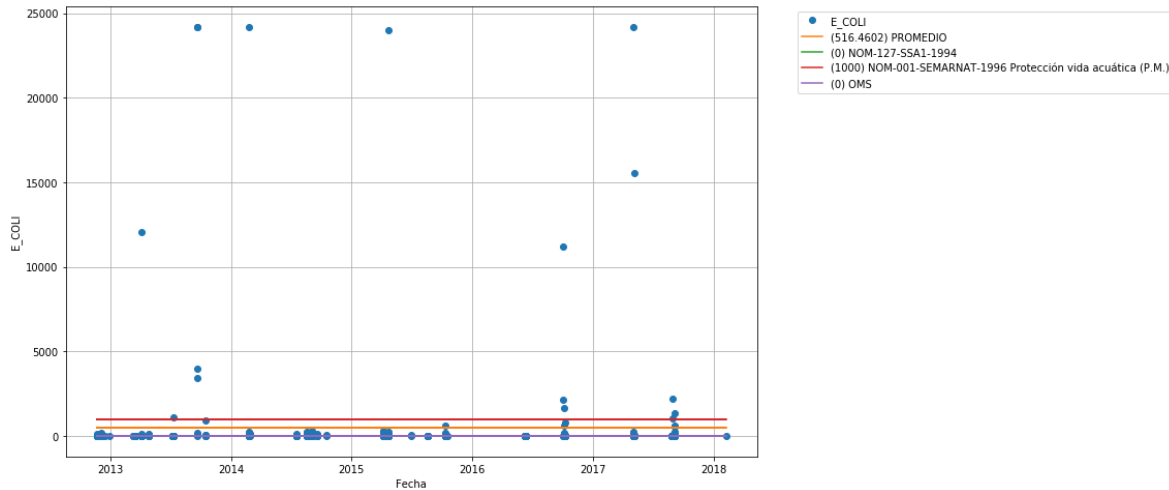
Figura 18. Concentraciones de Escherichia Coli obtenidas durante el periodo de medición, comparado con las normas disponibles para el parámetro
