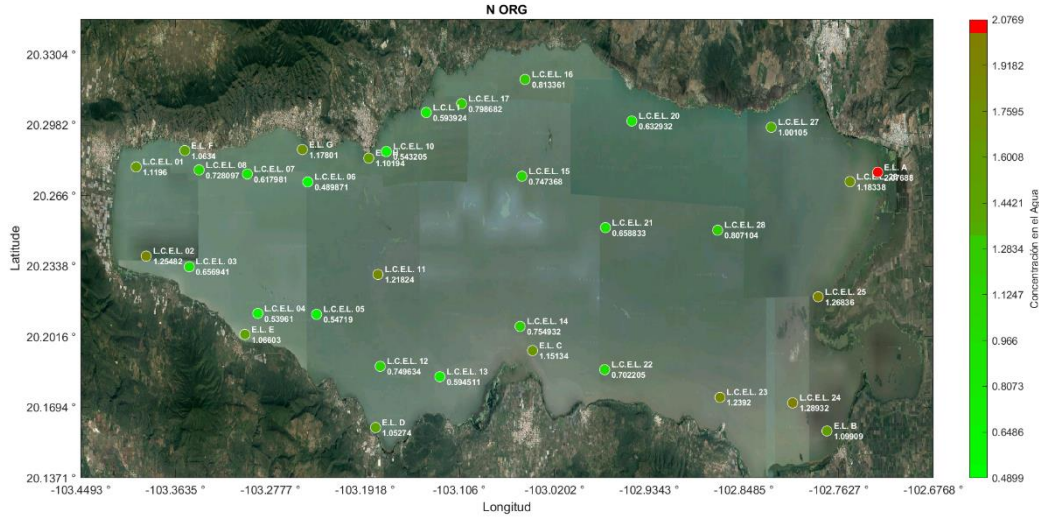
Figura 35. Localización de concentraciones de N_{ORG} .
