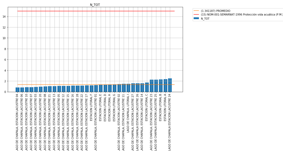
Figura 37. Valores promedio de la concentración de Nitrógeno total por estación de monitoreo comparado con las normas disponibles.
