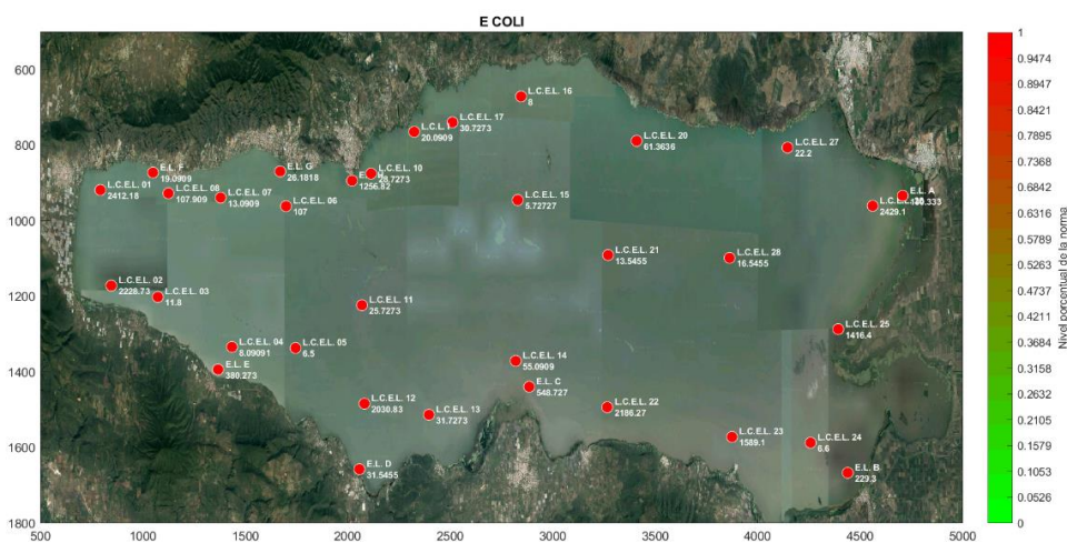
Figura 61. Concentraciones de E_COLI con referencia en la norma NOM-127-SSA1-1994.
